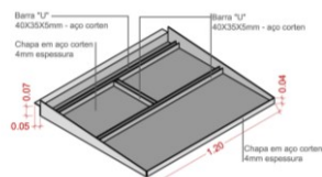
Axonometria - Vista inferior Escala 1:20
