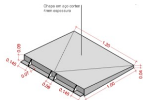
Axonometria - Vista superior Escala 1:20
