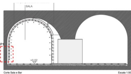
Corte Sala e Bar Escala 1:50
